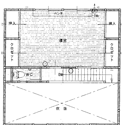
2階 間取り図
