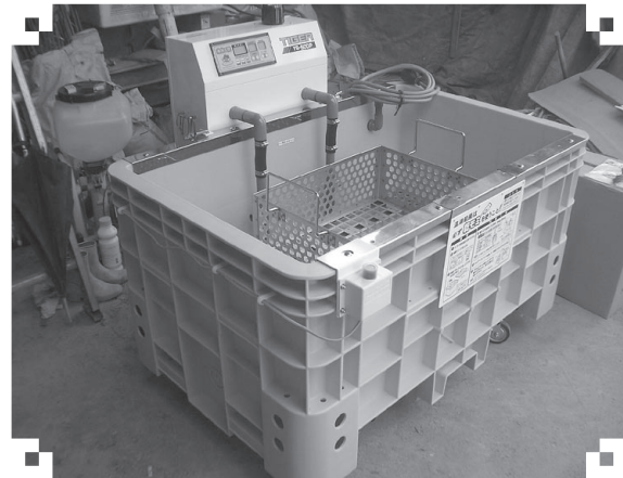
温湯消毒機
